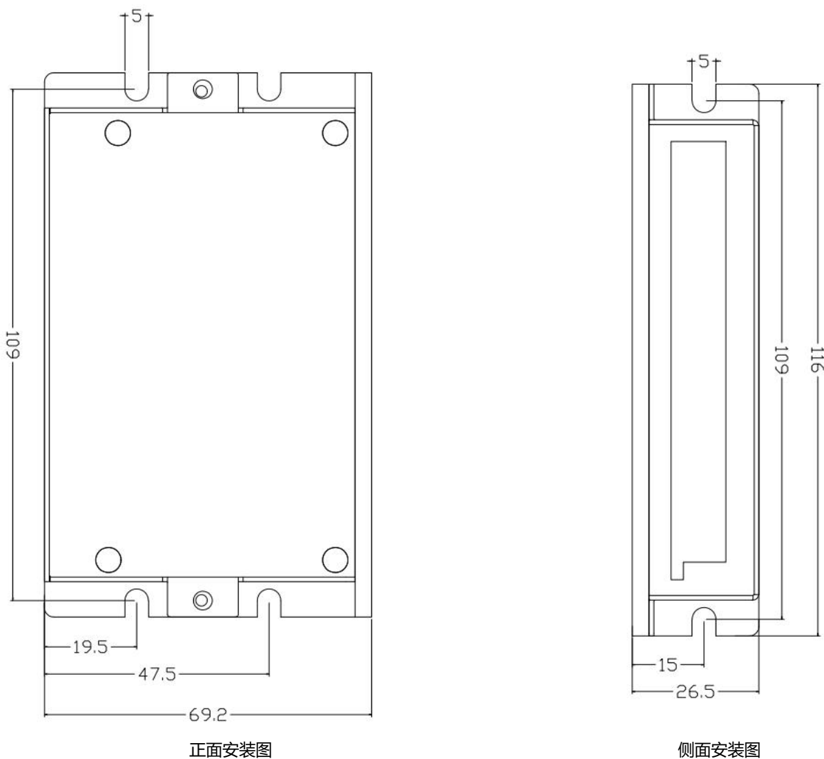
图 1 安装尺寸图 (单位: mm)
