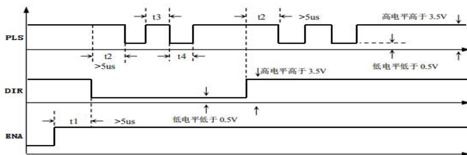
图 3 控制信号时序图
