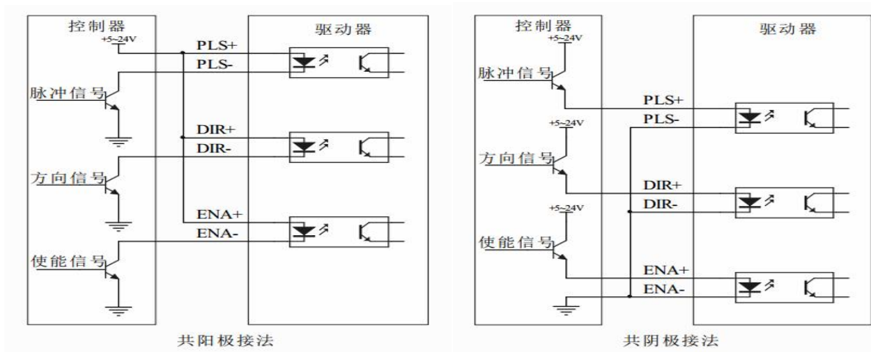
图 2 输入接口电路
